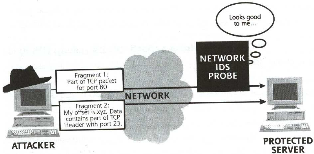
شکل (۶-۲۱) حمله به IDS مبتنی بر مکانیزم قطعات همپوشان (Fragment Overlap Attack)
