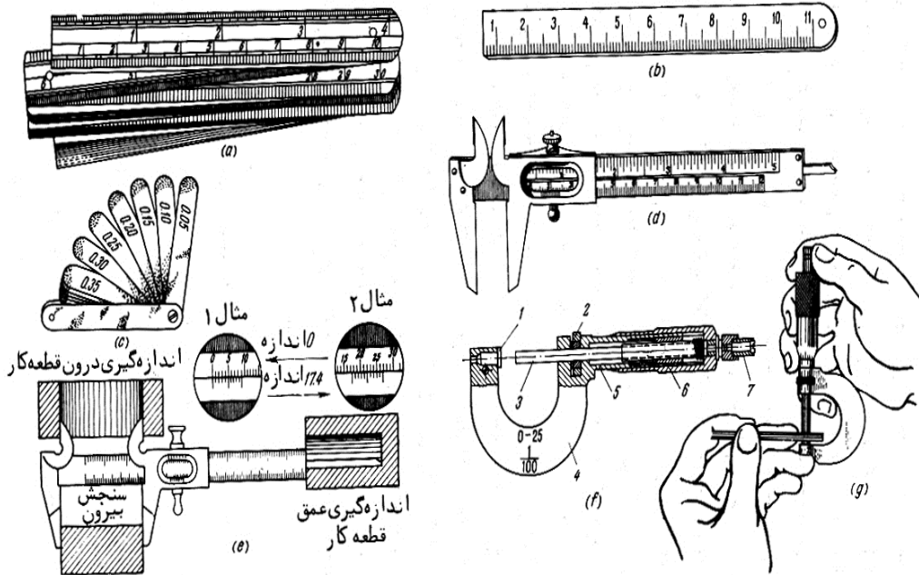
شکل (۵-۱): ابزار و ادوات اندازه گیری
