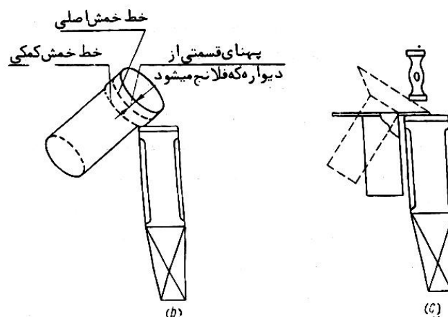
شکل (۵-۲۲): فلانچ کردن به خارج
