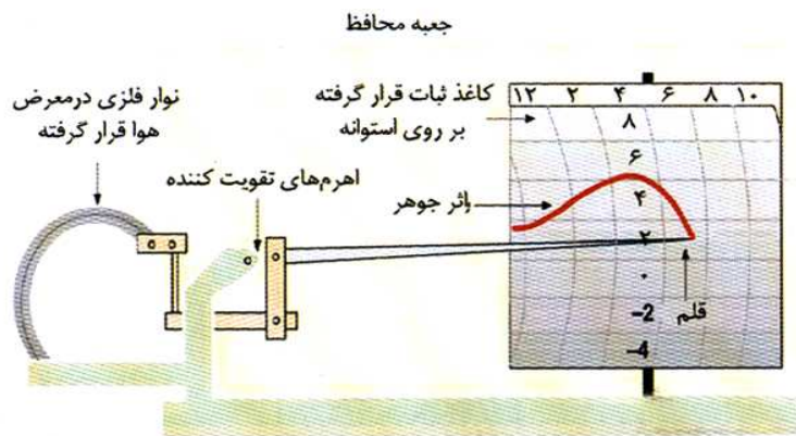
شکل (۲-۴): نمونه ای از یک دمانگار با یک گرما سنج فنری دو فلزی
