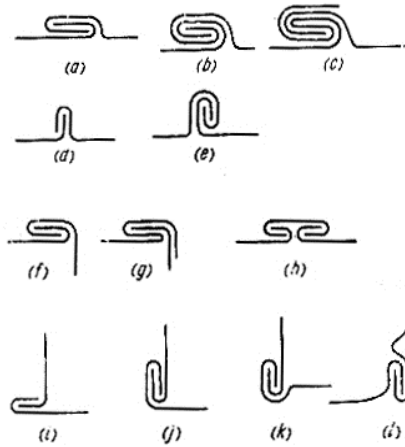
شکل (۵-۲۱): انواع اتصالات درز
